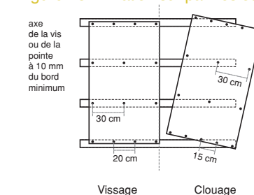
Figure 46 : Fixation sur pannes ou fourrures métalliques
